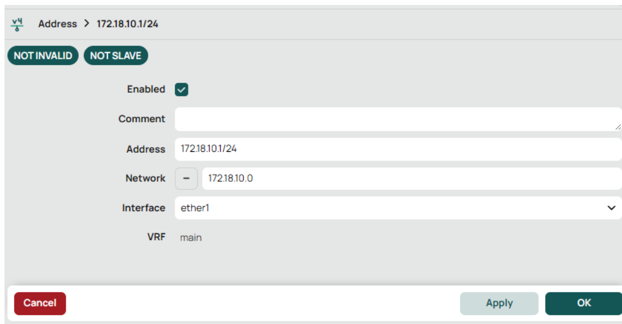
Ilustración 72 Router Mikrotik - IP interfaces 2
