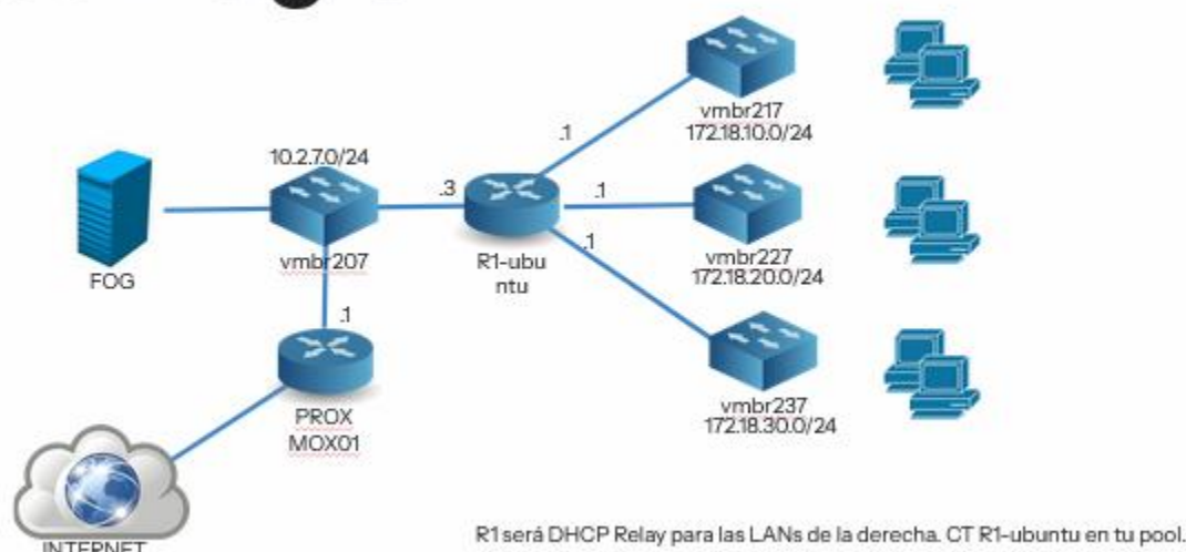
Ilustración 1 Diagrama de Red
