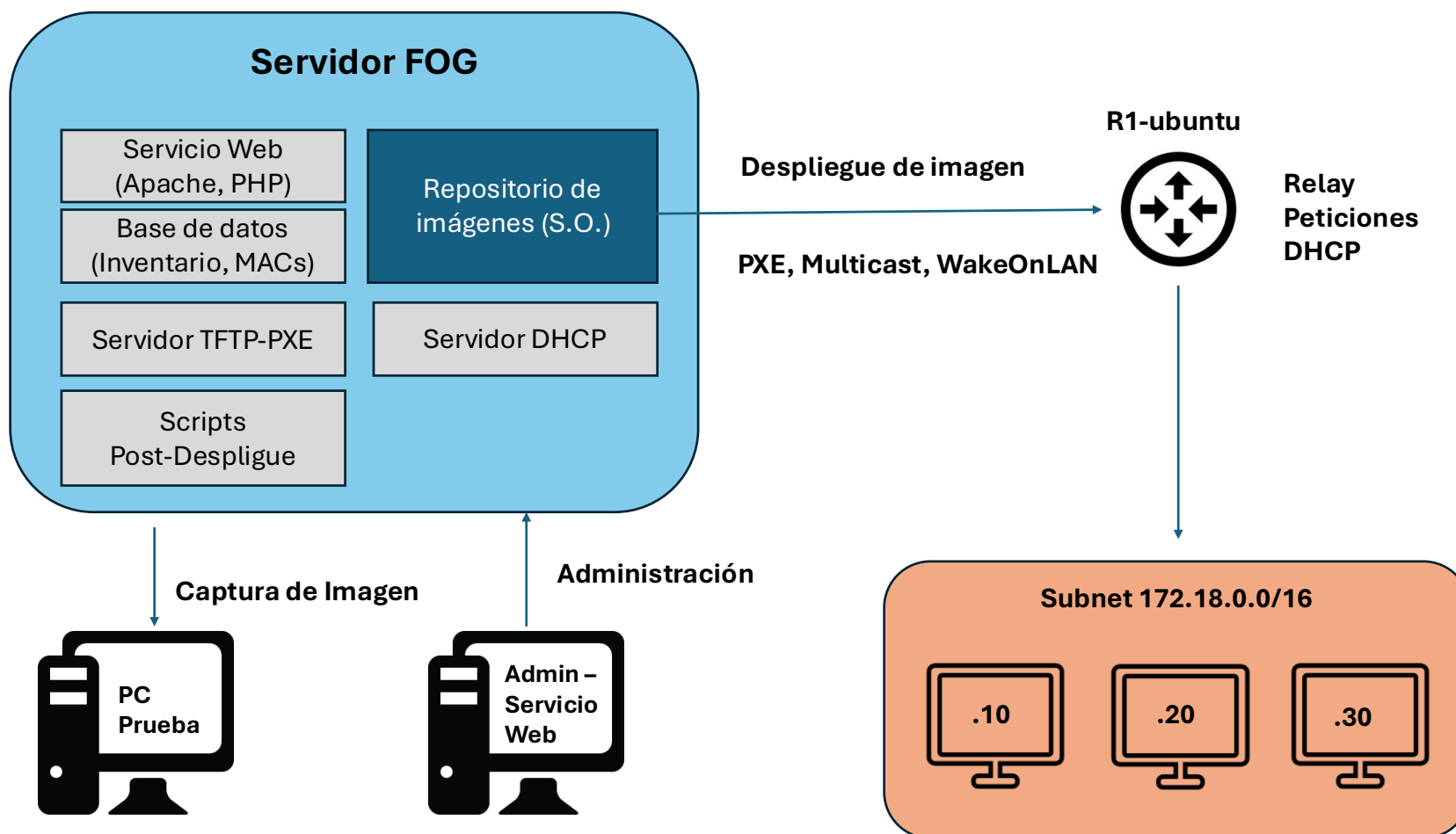
Ilustración 2 Diagrama conceptual del Servidor FOG y su funcionamiento
