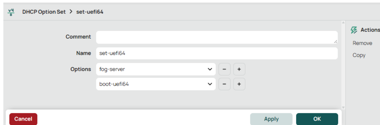
Ilustración 103 Router Mikrotik - DHCP-Server - Options Sets 2
